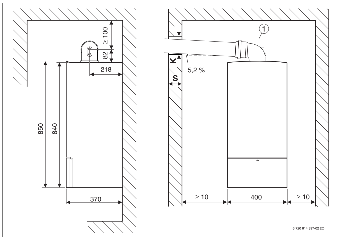
Фиг. 6 Димоотвод Ø 60/100 mm
