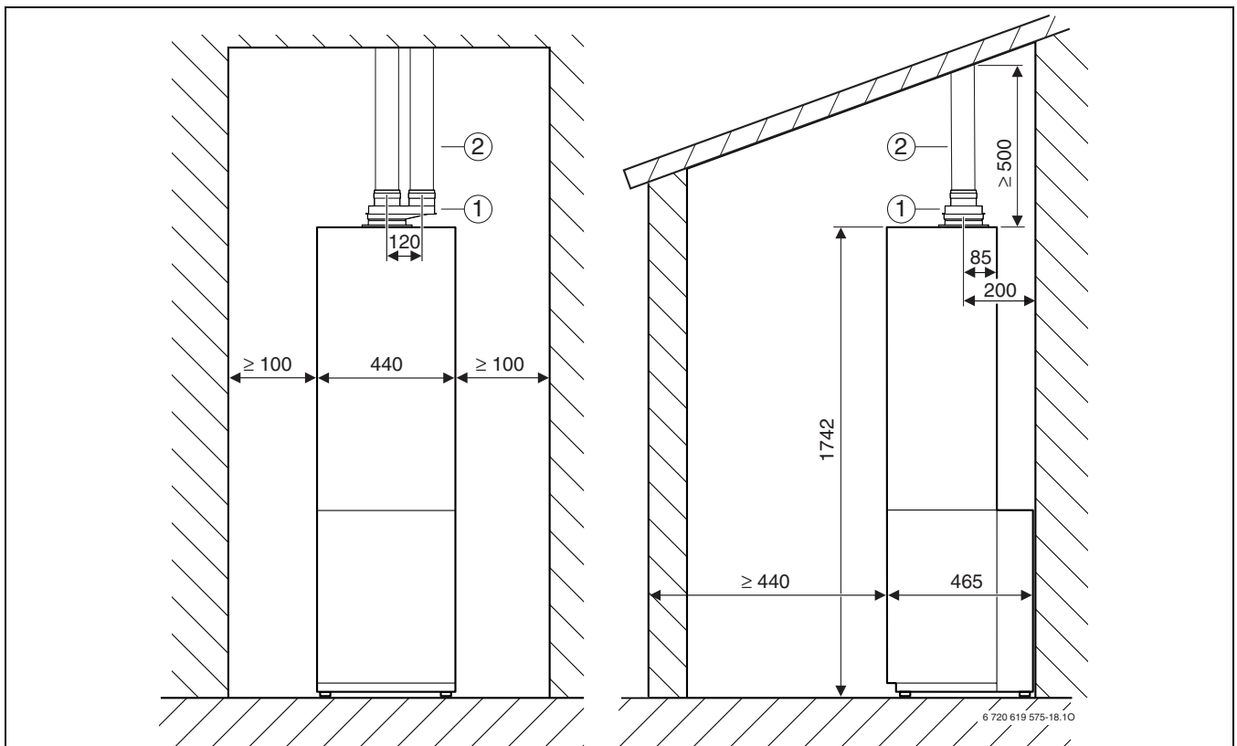
Фиг. 20 Ø 80/80 mm, наклонен покрив
