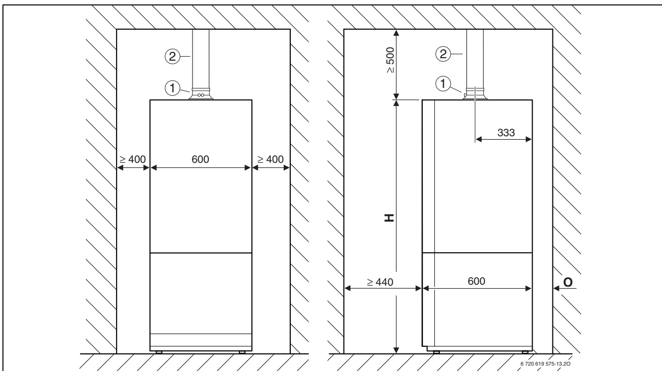
Фиг. 15 Ø 60/100 mm, плосък покрив
