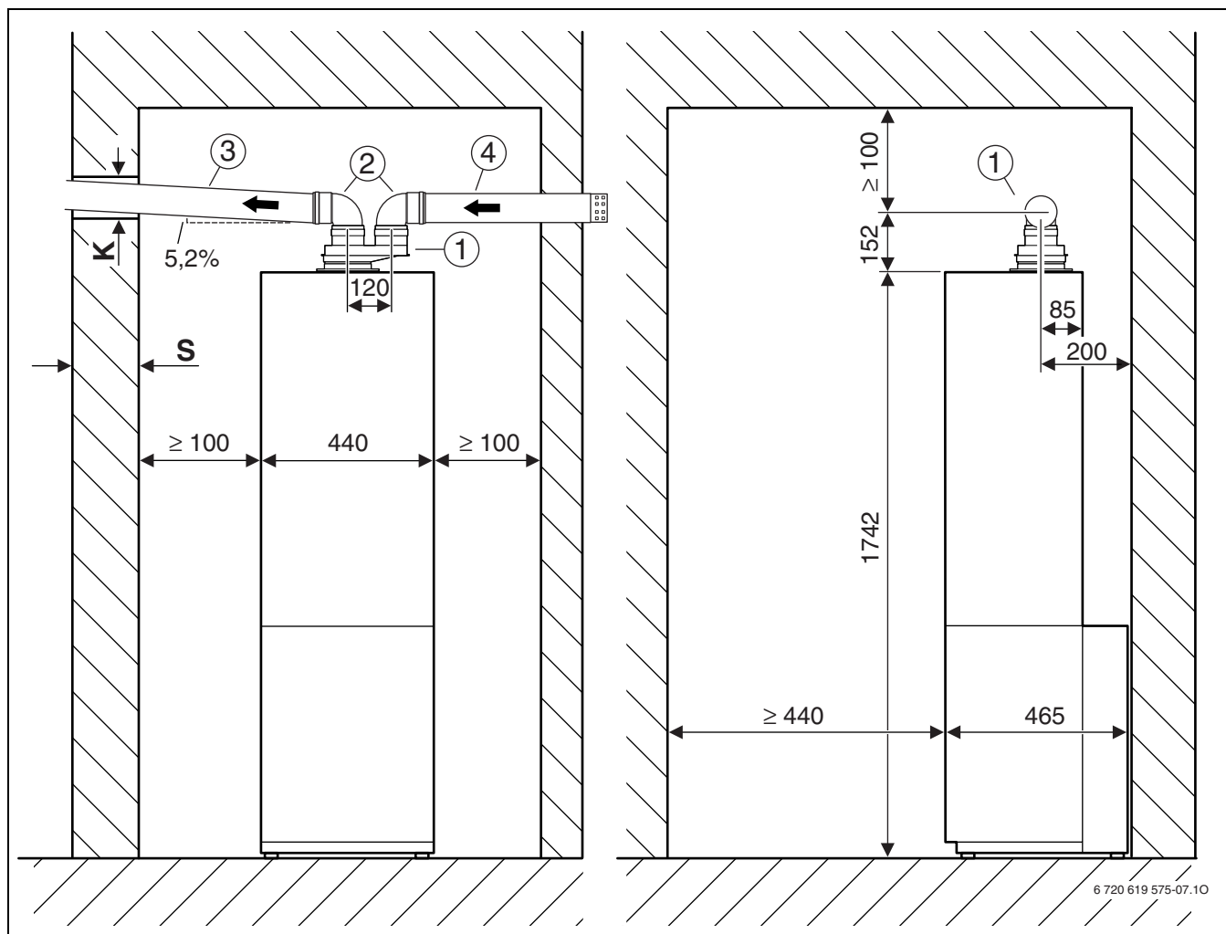
Фиг. 17 Ø 80/80 mm
