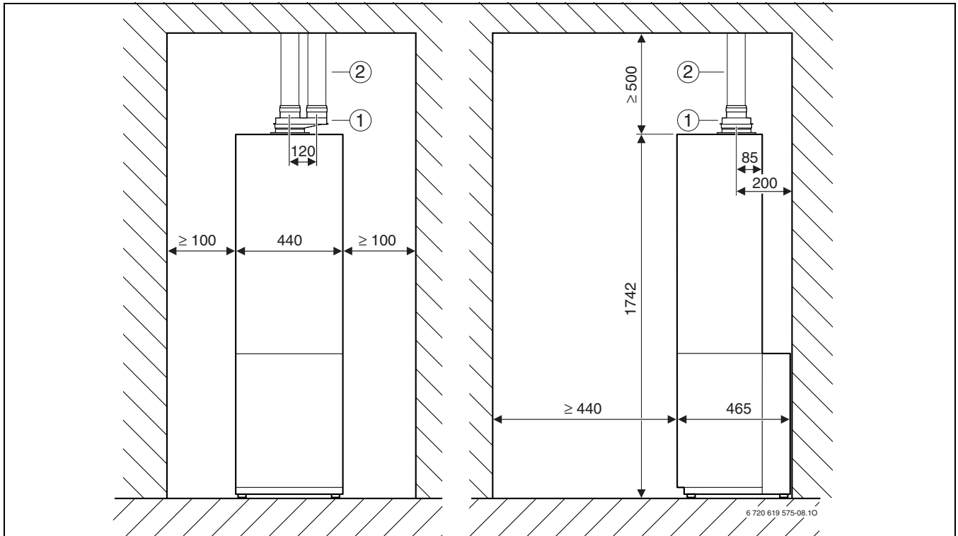
Фиг. 19 Ø 80/80 mm, плосък покрив
